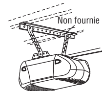
FIGURE 2 Plafond fini
