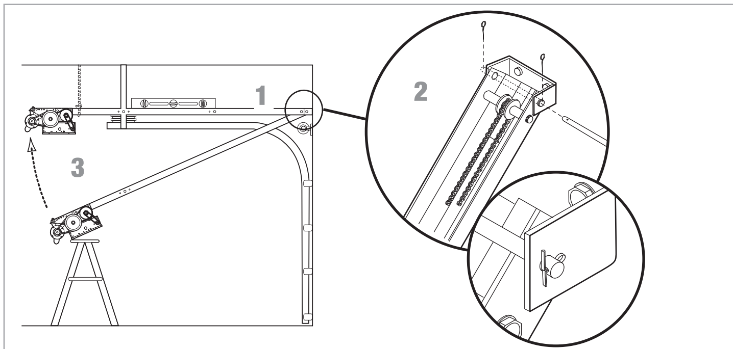
Goupilles fendues (2)
