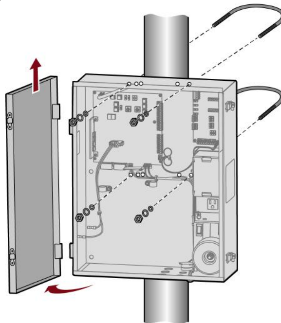
Montage mural ou sur colonne
