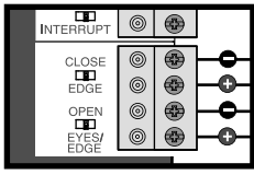
Control Board Carte logique Tablero de control
